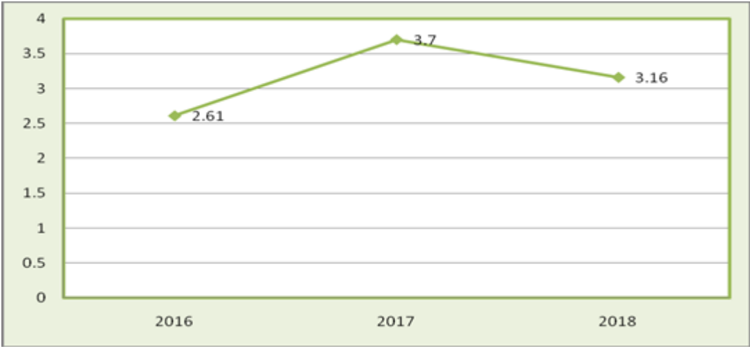
Gambar 3- 3. Inflasi Tahun 2016-2018
